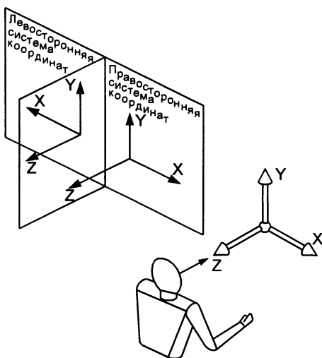
Рисунок 1 — Координатная система электронной модели изделия
